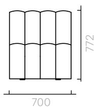
Straight Module
