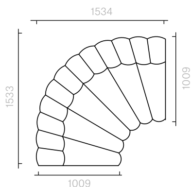
Corner Module
